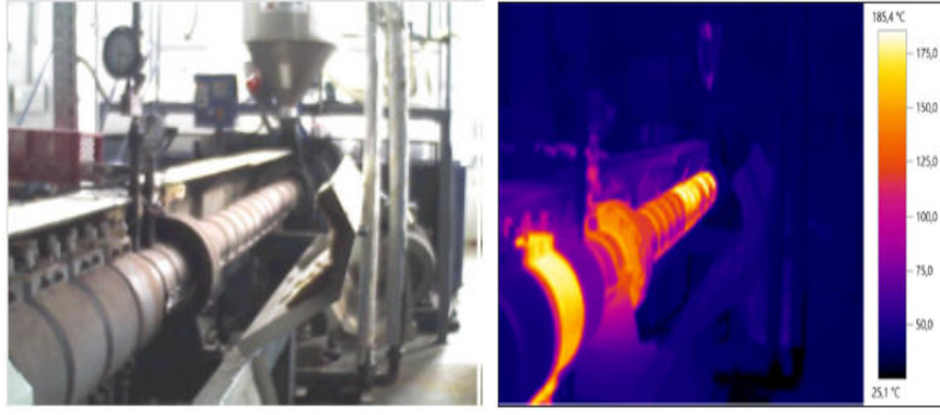
Ekstruder termal kamera görüntüsü ve Enerji kayıplarının tespiti
