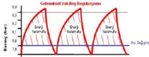
Kompresör yükte boştta çalışma çalışma grafiği
