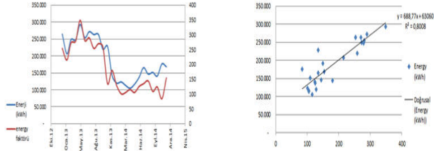
2012-2015 yılları arası Enerji Kullanımı ve Enerji kullanımına etki eden faktör trendleri Enerji kullanımlarına ait regresyon analizi ve grafiği
